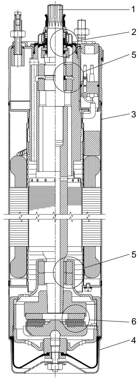
Fig. 16 MS 4000
