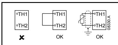
Figure 4-3 Raccordement des sondes thermiques moteur
