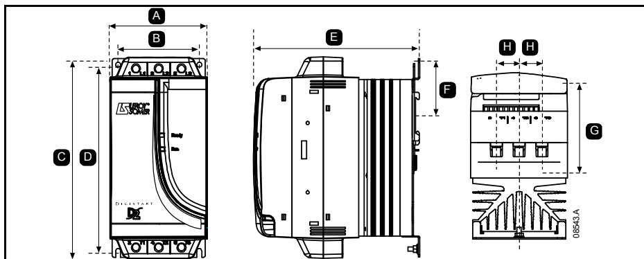
Figure 3-1 Dimensions de l'appareil
