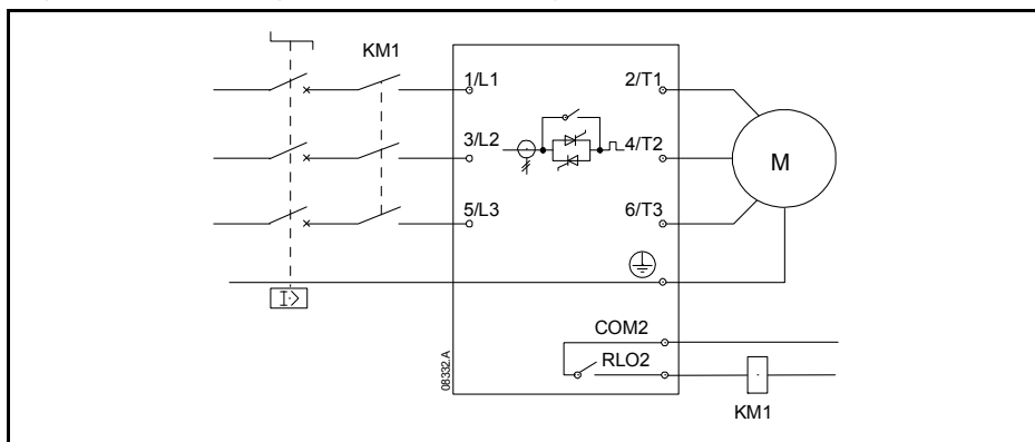
Figure 4-5 Démarreur progressif avec disjoncteur magnéto-thermique et contacteur principal
