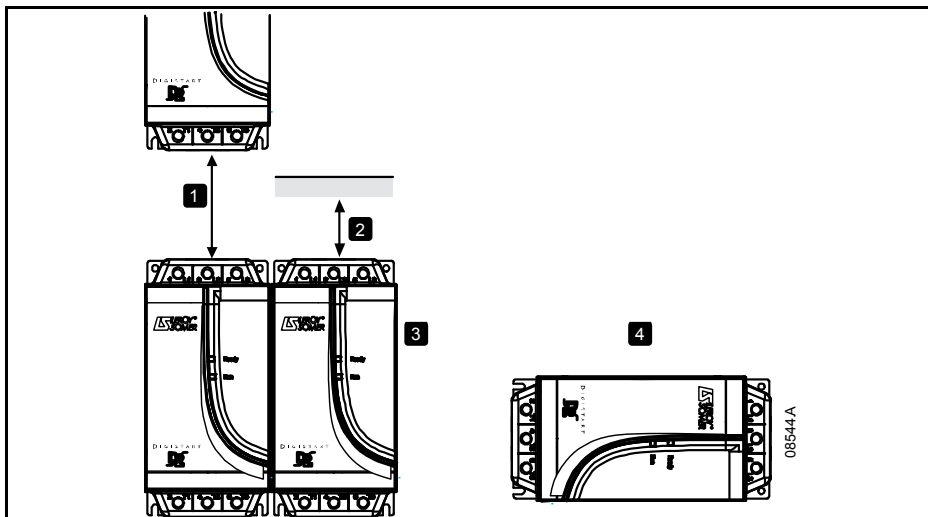
Figure 3-2 Espaces d'installation
